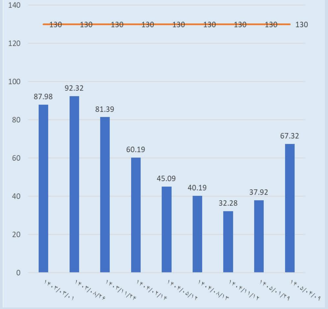
غلظت غبار الکترو فیلتر اصلی خط ۱ پری هیتر (mg/nm 3 ) سال ۱۴۰۳-۱۴۰۴-۱۴۰۵
