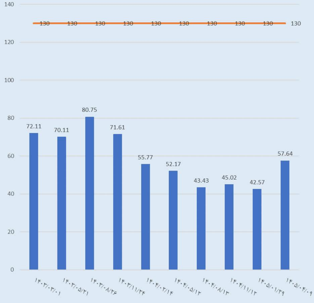
غلظت غبار الکترو فیلتر اصلی خط ۲ پری هیتر (mg/nm 3 ) سال ۱۴۰۳-۱۴۰۴-۱۴۰۵
